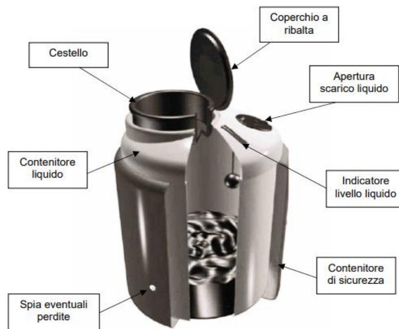
Fig.2 - sezione del contenitore
